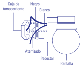
DIAGRAMA ELÉCTRICO (B) Cable blanco: Neutro (N) Cable negro: Línea (⊕) Cable de cobre: Tierra
